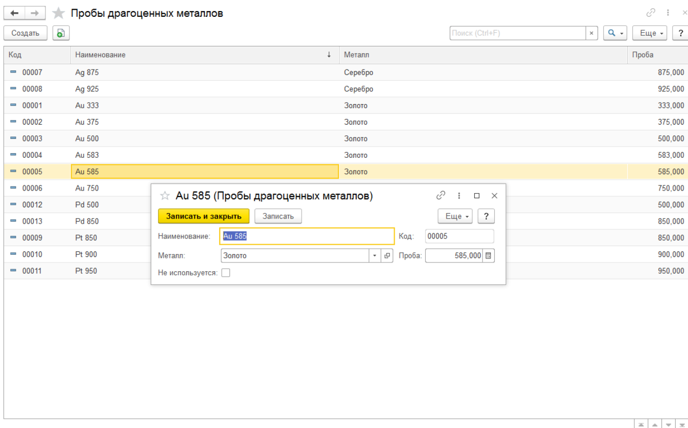
Рис. 4.10. Справочник Пробы.
