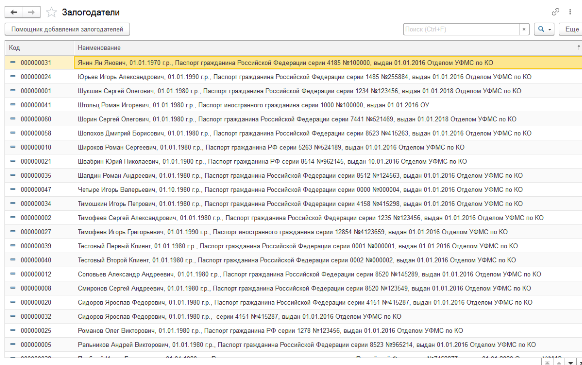
Рис. 4.5. Залогодатели.
