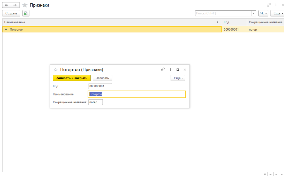
Рис. 4.9. Справочник Признаки.
