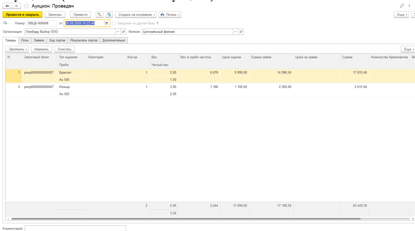
Рис. 1.12. Документ «Аукцион».
