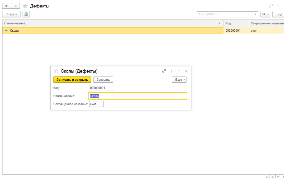
Рис. 4.3. Справочник Дефекты.
